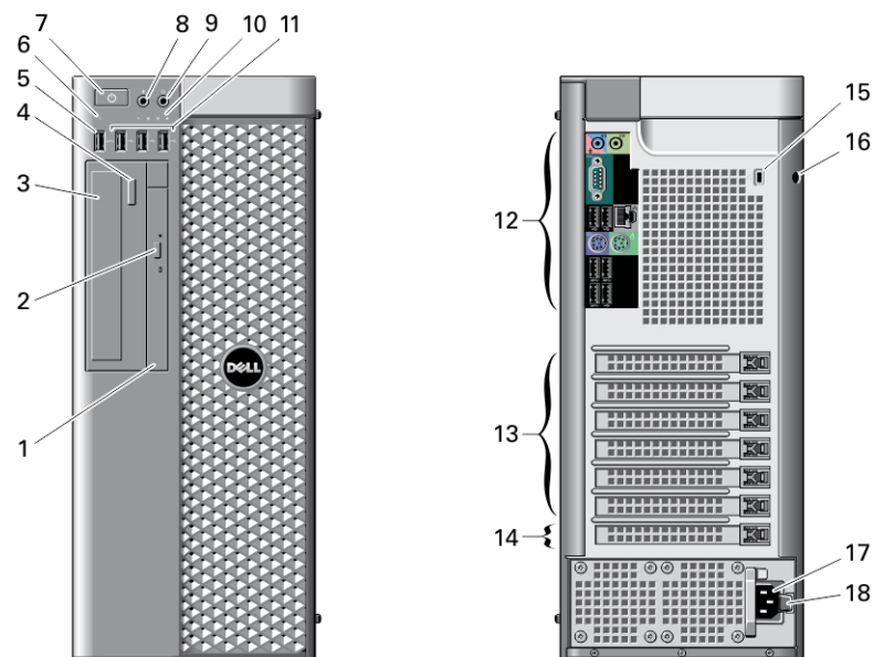
Figur 1. Fram- och baksida av T3610/T5610
